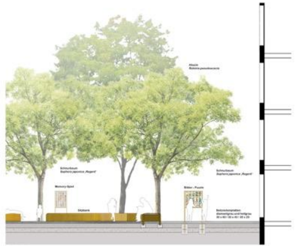
Detailschnitt M 50
